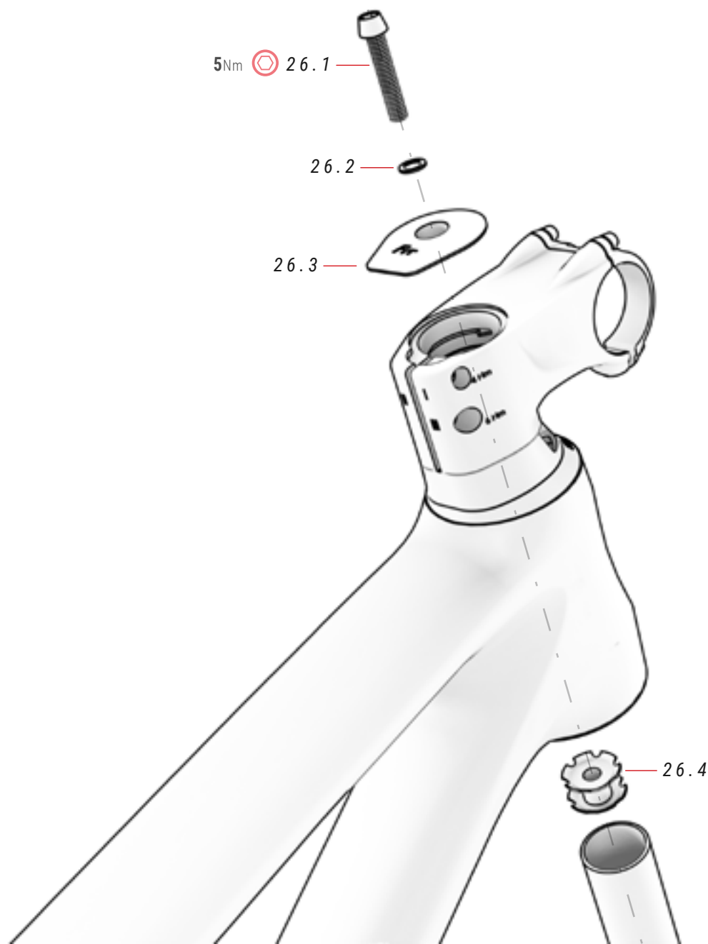
26 COVER EN SPIN ref.: 363297300
